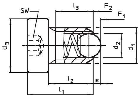
Größe M4-M5
