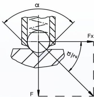
Standard-Federkraft
