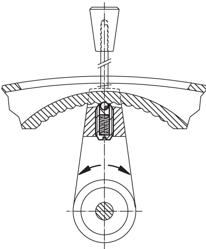
Standard-Federkraft
