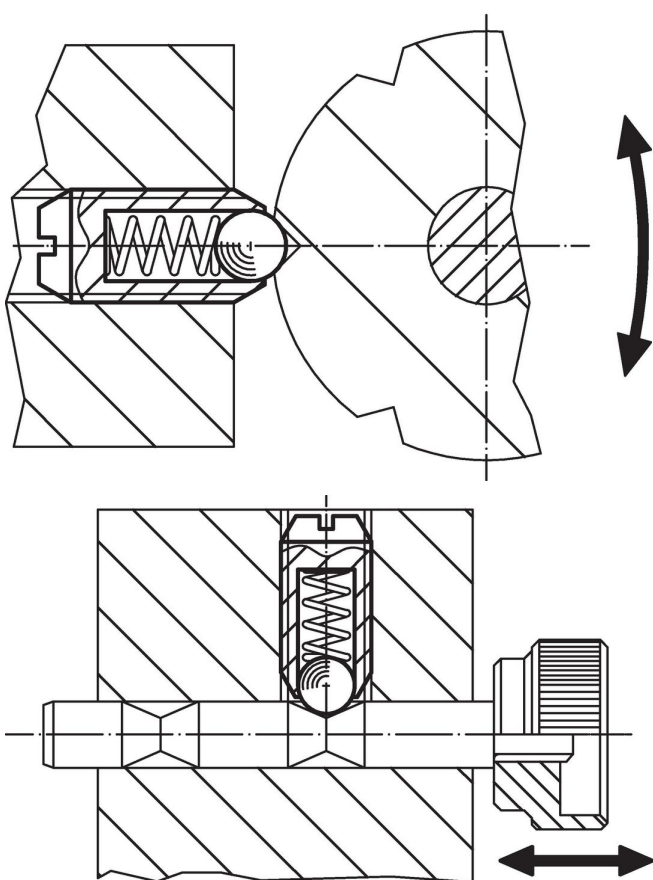
Standard-Federkraft
