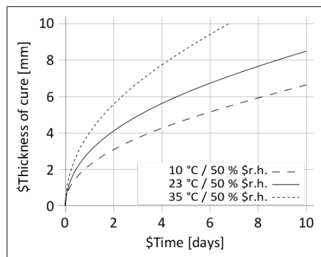
Diagramm 1: Durchhärtengeschwindigkeit Sikaflex®-554
