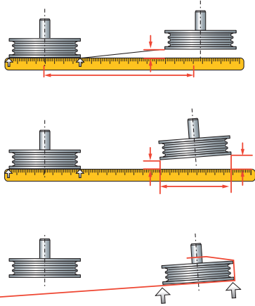
Messung des Parallel- und Winkelversatzes mit Hilfe eines Lineals oder einer Schnur.
