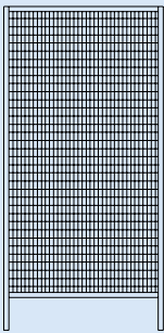
Wandelemente in 4 Breiten, Höhe: 2000 mm, Bodenfreiheit 200 mm
