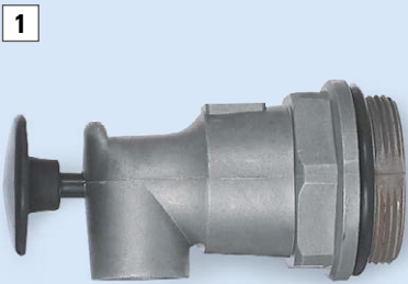
Aluminiumzapfhahn 2", federbelasteter Betätigungsknopf
