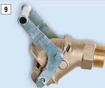
Messingzapfhahn 2", mit Verschlussplatte mit PTFE-Dichtung
