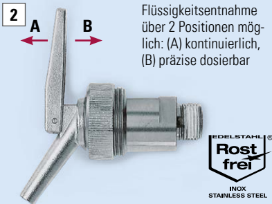
Edelstahlfeindosierhahn 3/4"
