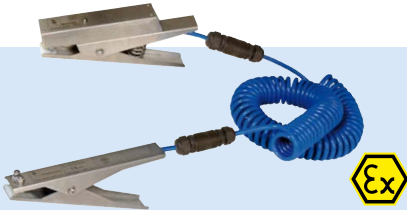
Typ EZ mit 2 Zangen. Mobil und sicher - verbindet 2 Behälter oder 1 Behälter, Tankfahrzeug etc. mit Erdungspunkt und zeigt über eine LED an, wenn beide Zangen sicheren Kontakt haben.
