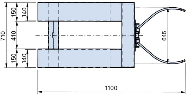
Draufsicht: Fassklammer Typ FK
