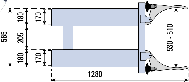
Draufsicht: Fassklammer Typ SK
