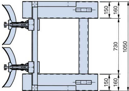
Draufsicht: Fassgreifer SH 2.
