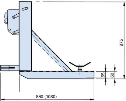
Seitenansicht: Fassgreifer SH 1 und SH 2.
