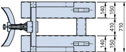
Draufsicht: Fassgreifer SH 1.
