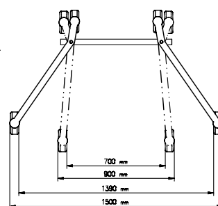
Maße Fahrwerk eingeklappt / ausgeklappt.
