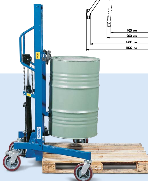
Maße Fahrwerk eingeklappt / ausgeklappt.
