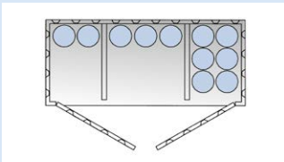
Bestückungsbeispiel MDC 210
