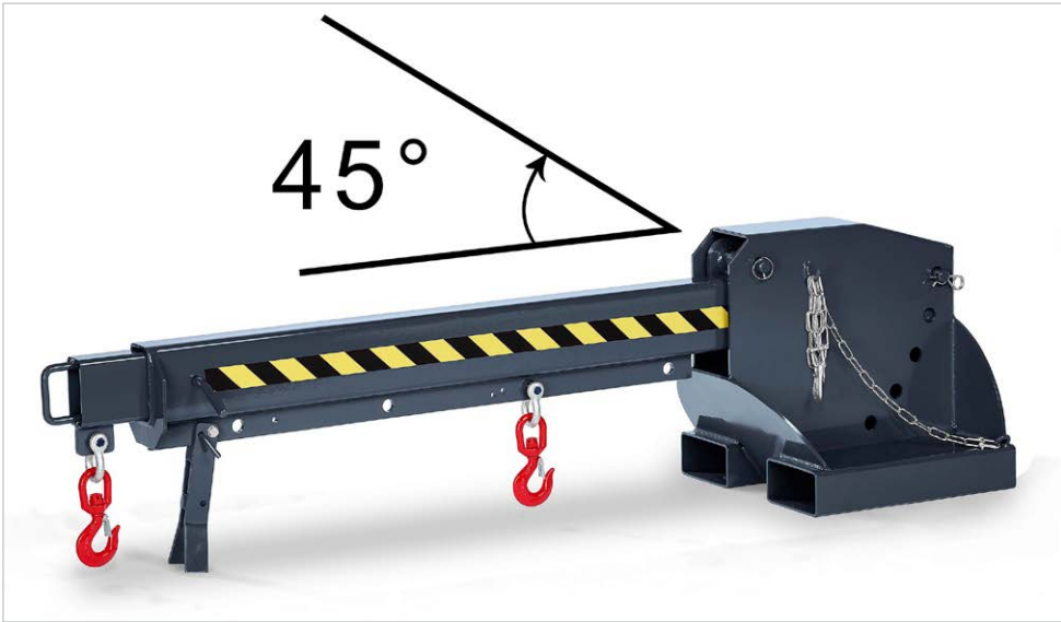
Kranarm, auszieh- und höhenverstellbare Ausführung (6-fach ausziehbar, 5-fach höhenverstellbar bis 45°)
