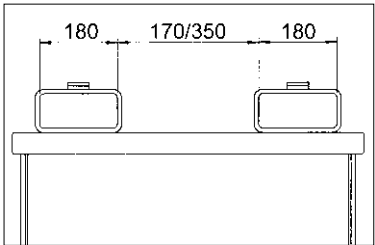
Maße Gabeltaschen (mm), 350 mm bei 1000 L
