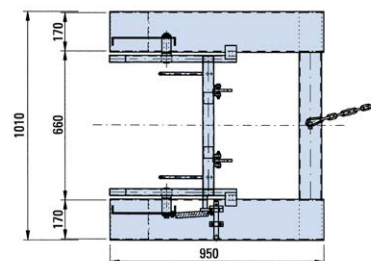
Draufsicht MT 240 Maße in mm
