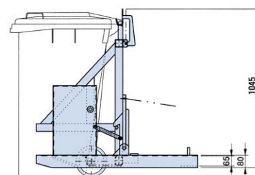
Seitenansicht MT 240 Maße in mm
