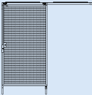
Schiebetür mit Laufschiene und Anschlagpuffern. Verriegelung durch Magnetverschluss, mit Klinkengriff
