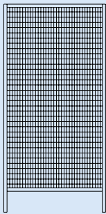
Wandelemente in 4 Breiten, Höhe: 2000 mm, Bodenfreiheit 200 mm
