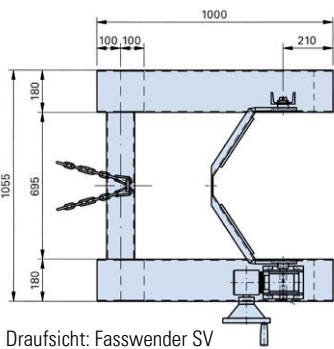
Draufsicht: Fasswender SV
