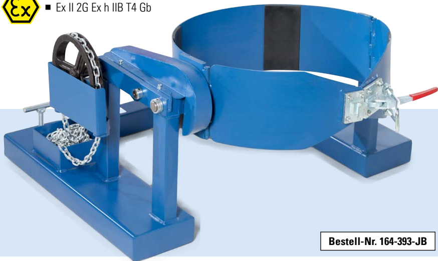
Bedienung mittels Endloskette vom Fahrersitz.
