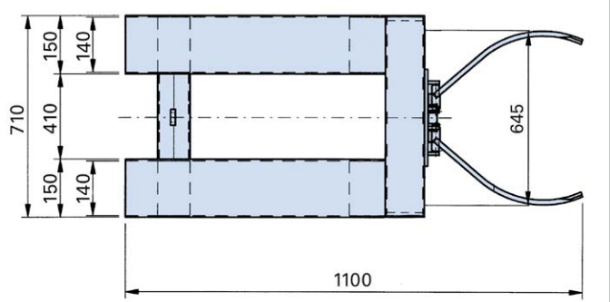
Draufsicht: Fassklammer Typ FK
