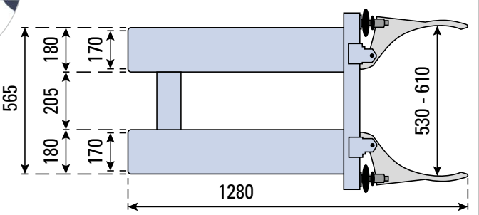
Draufsicht: Fassklammer Typ SK
