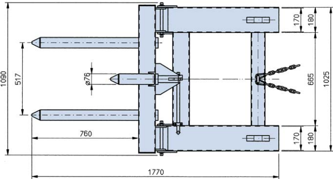
Draufsicht: Fassgreifer RLN.
