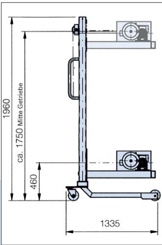
Seitenansicht: Fassheber mit Fasswender 180°
