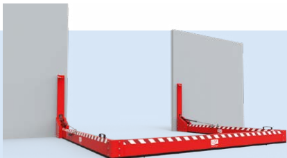
Schwenkbare Laderampenbarriere für Türen/Tore bis zu einer lichten Breite von bis zu 3500 mm
