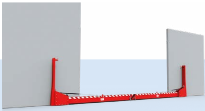
Schwenkbare Doppelbarrieren für Türen/Tore mit einer lichten Breite von 4000 bis zu 7000 mm
