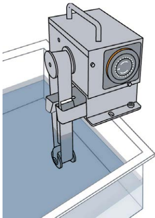
Typische Anwendung: Öl-Bandskimmer mit Montagefuß, montiert auf dem Rand eines Behälters
