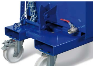
Detailabbildung: Ablasshahn
