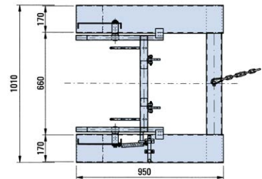
Draufsicht MT 240 Maße in mm
