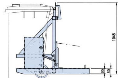
Seitenansicht MT 240 Maße in mm
