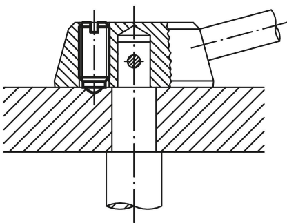
Schalthebelarretierung
