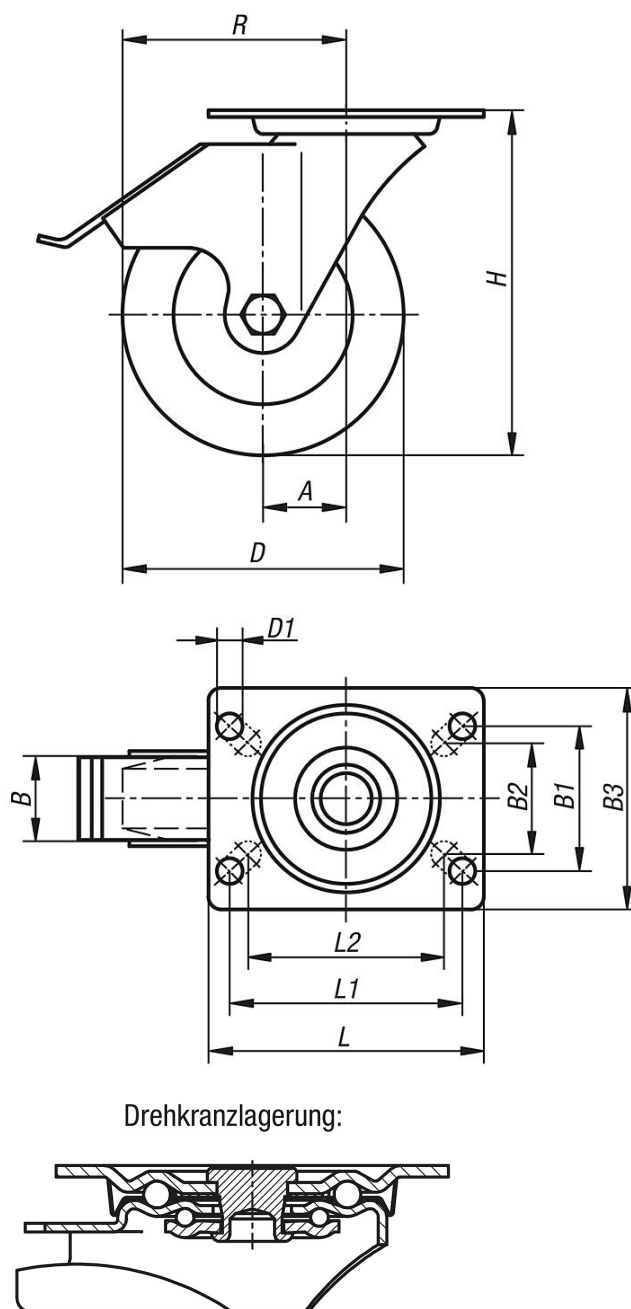
Lenkrolle mit „stop-fix“
