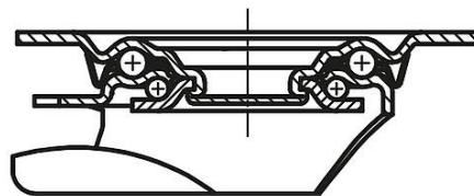
Drehkranzlagerung: Anschraubplatte
