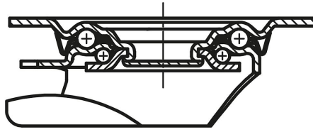
Drehkranzlagerung:
