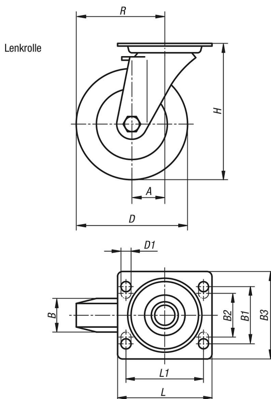
Drehkranzlagerung bis R1 = 125
