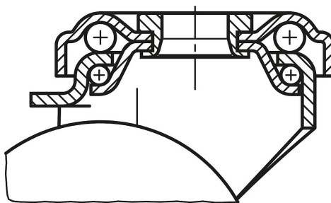
Drehkranzlagerung:
