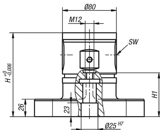
Fuß mit Langloch
