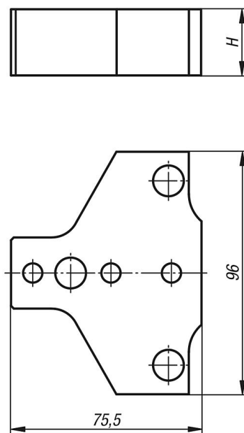
Adaptererhöhung für feste Seite
