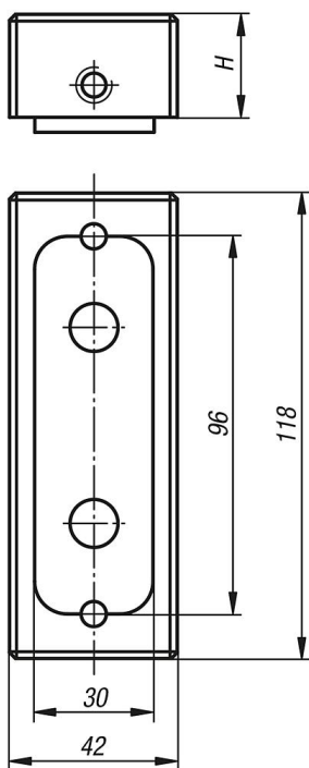
Adaptererhöhung für bewegliche Seite
