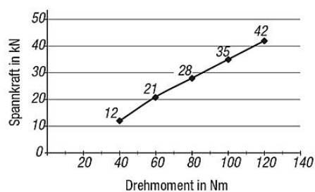
Spannkraft 5-Achs-Spanner
