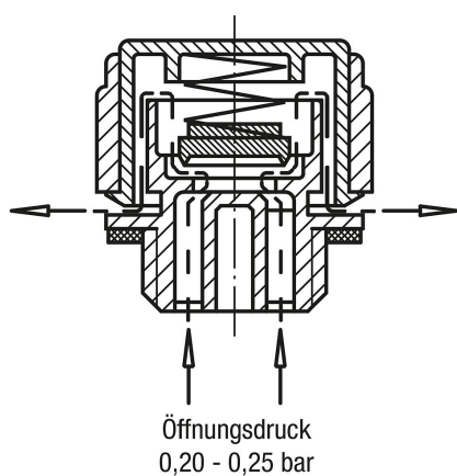
Funktionsprinzip
