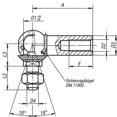
Form CS mit Sicherungsbügel
