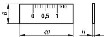
Nonius
