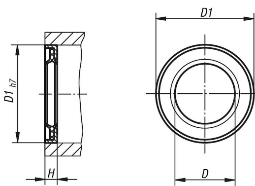
Ausführung geschlossen
