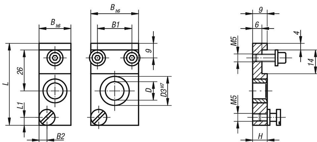
Bohrbuchsenträger
