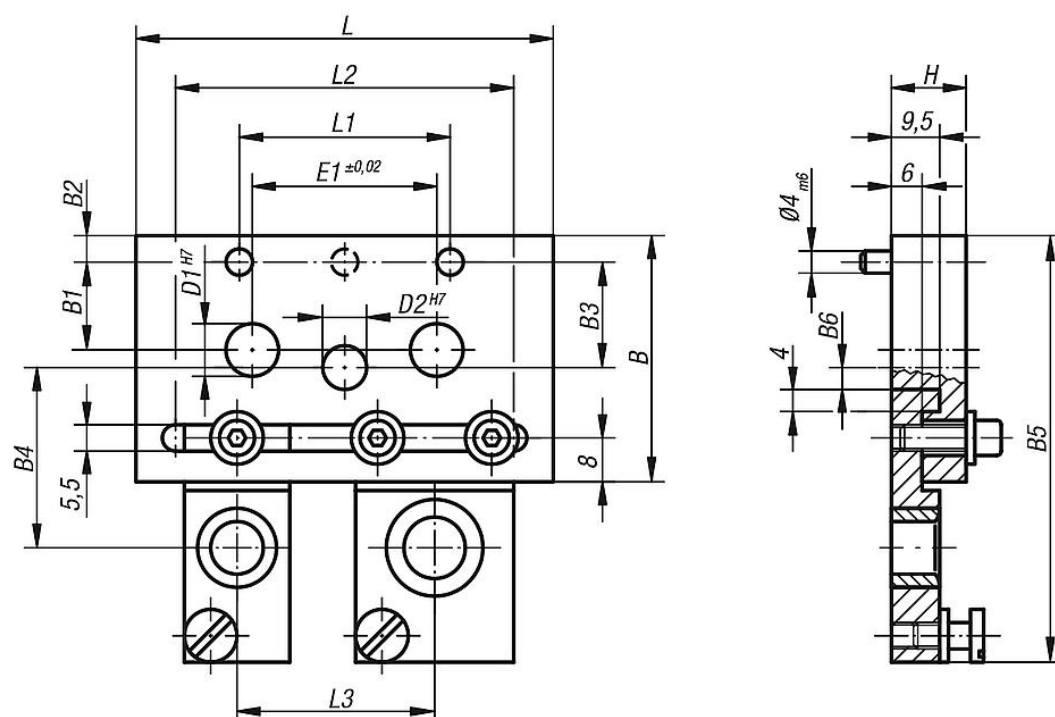
Bohrbuchsenträger-Platte
