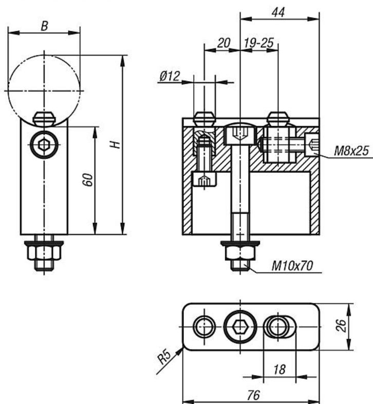
Spannschema Halter:
