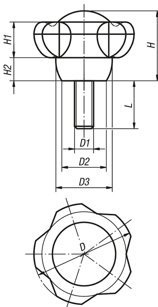
Klemmgriff mit Außengewinde
