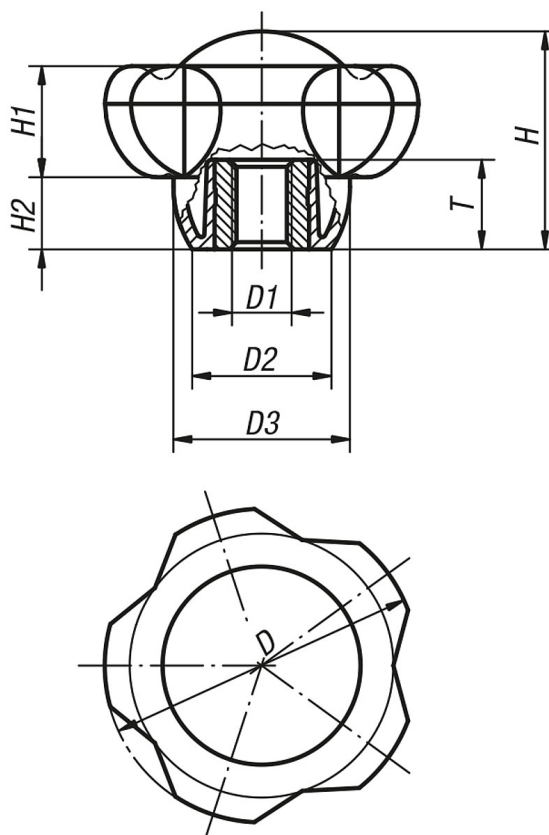
Klemmgriff mit Innengewinde
