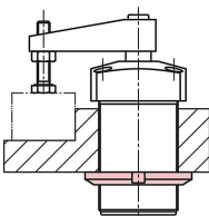
Mit einer Nutmutter von unten.
