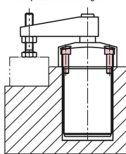
Mit vier Zylinderschrauben von oben.
