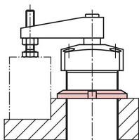
Mit einer Nutmutter von oben.
