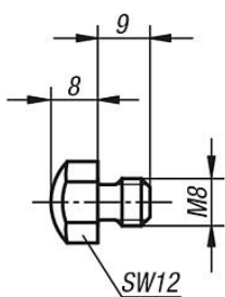
Druckstück
