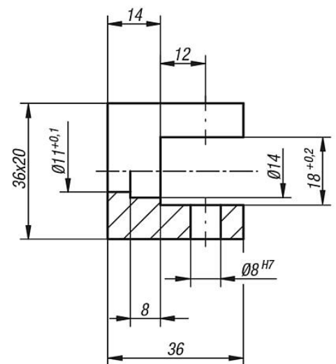
Gabelstück
