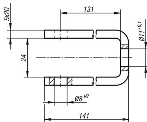
Zugbügel
