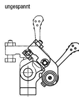
Spannen bearbeiteter Oberflächen
