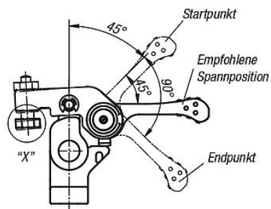
Spannen roher Oberflächen
