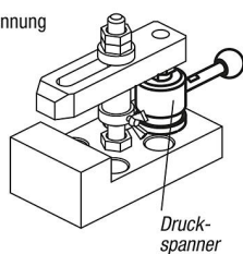
Horizontalspannung
