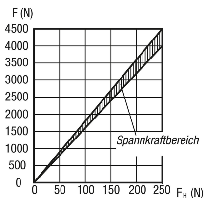
Kräfte diagramm
