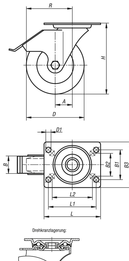
Lenkrolle mit „stop-fix“
