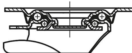
Drehkranzlagerung: Anschraubplatte
